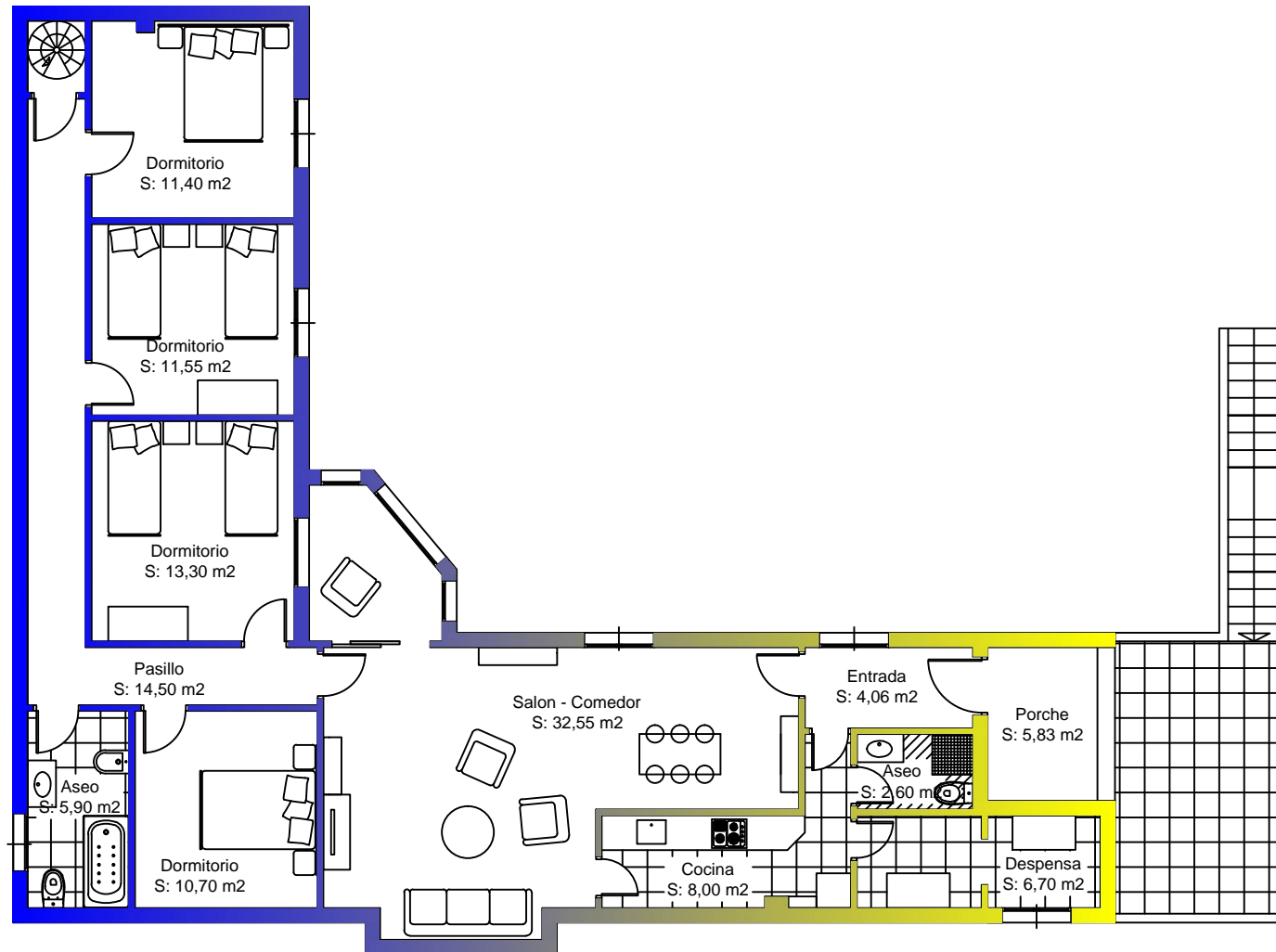
PLANTA PRIMERA ACTUAL
